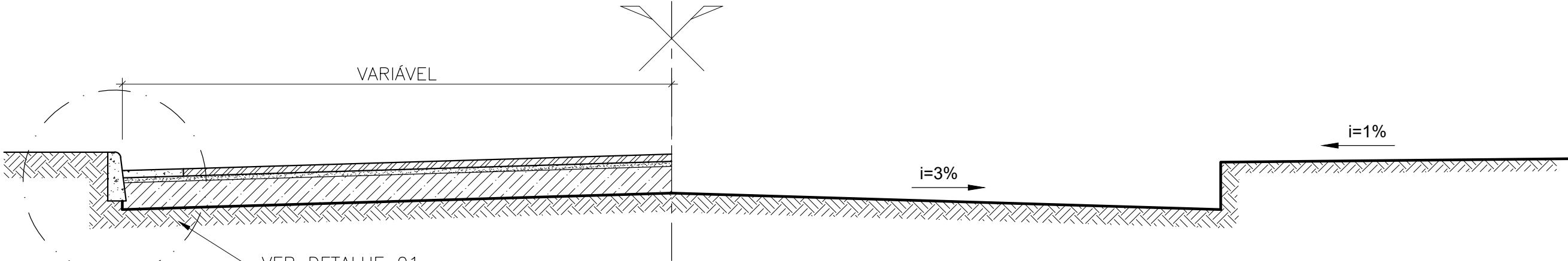
SEÇÃO TIPO – CORTE AA SEM ESCALA
