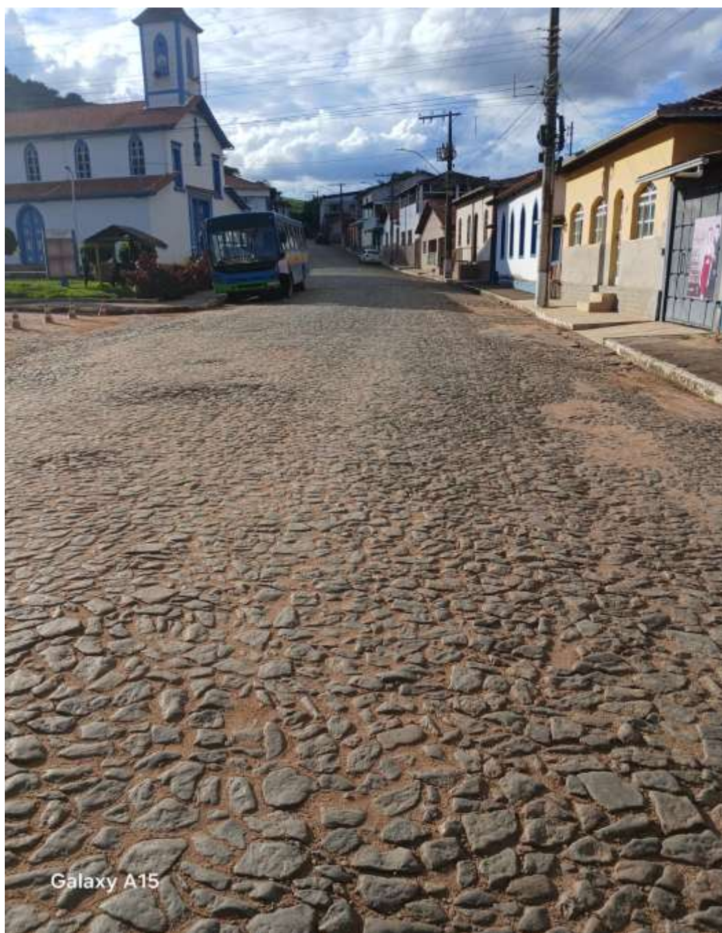
Foto 03 – Presença de falhas e perda de material de rejunte entre as pedras.
